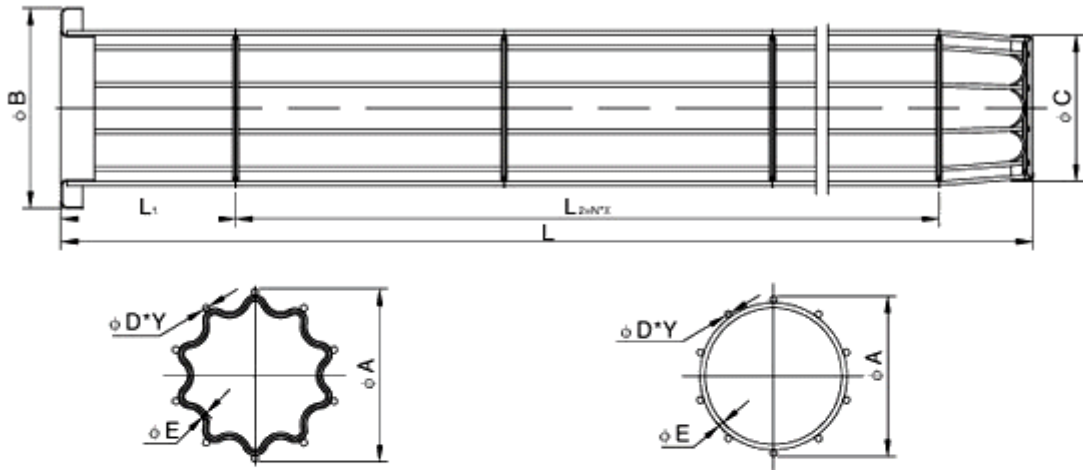
圖籠型濾袋框架外形圖
