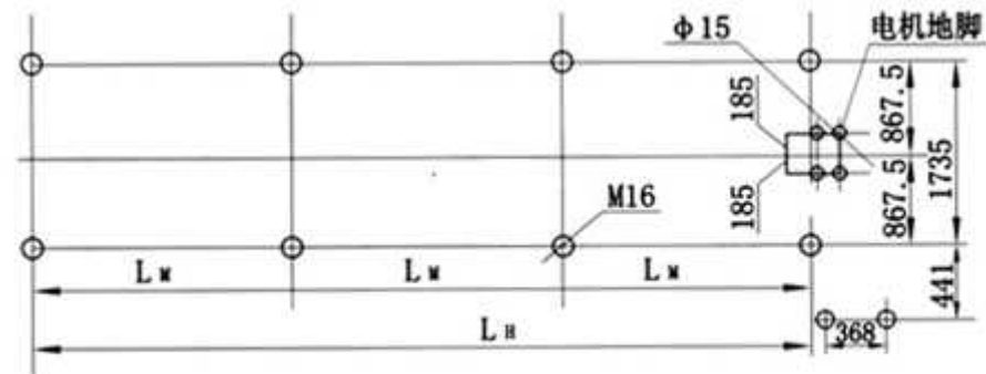
地脚尺寸
