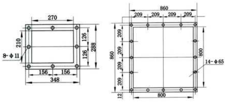
地脚尺寸
